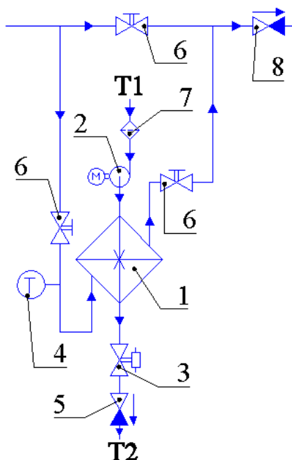
Гидравлическая схема
