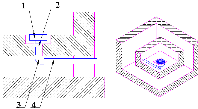
Рисунок 9 (установка сквозь дно)
