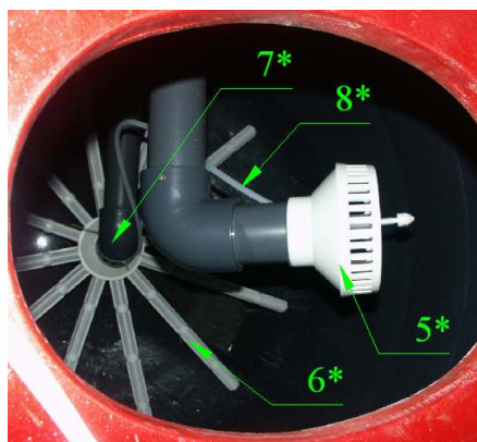
Детализовка «Позиции 2 Таблицы 2» (Обвязки фильтра Kripsol BD 90-110.B) изображена на рисунке 4. Рисунок 4
